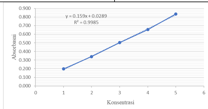
Gambar 1. Kurva Standar Kuersetin
