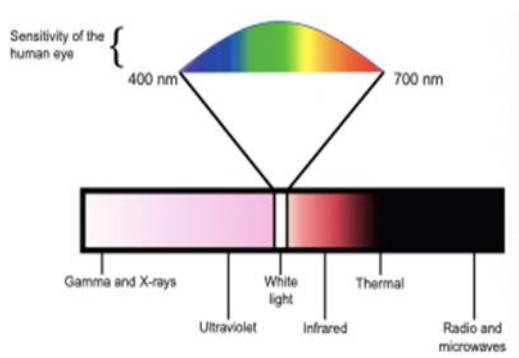
Gambar 2. Spektrum elektromagnetik
