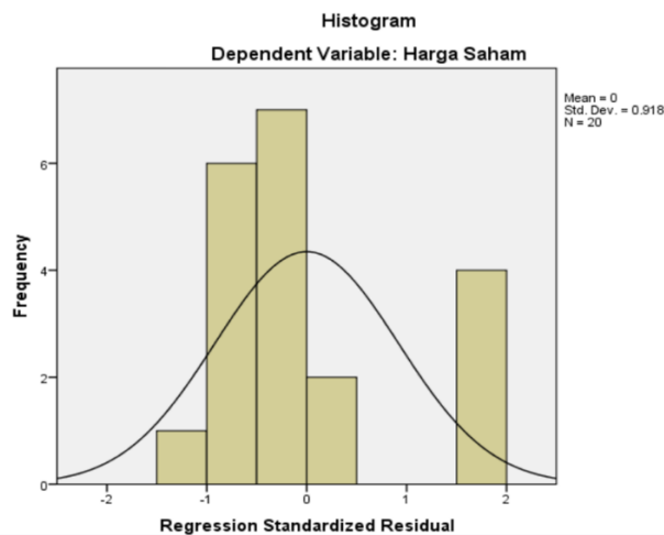
Gambar 3 Grafik Histogram
