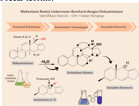
Gambar 1. Mekanisme Reaksi Liebermann-Burchard dengan Deksametason
