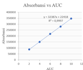
Gambar 3. Kurva Baku Parasetamol
