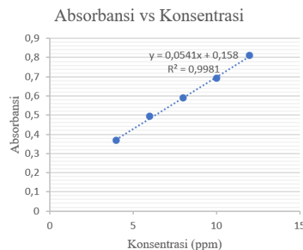
Gambar 2. Kurva Baku Jamu Deksametason
